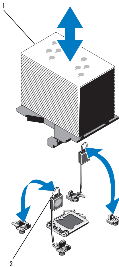
图 3-23. 安装和卸下散热器
