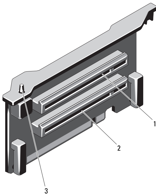
图 6-5. PCIe 扩充卡提升板 2 组件
