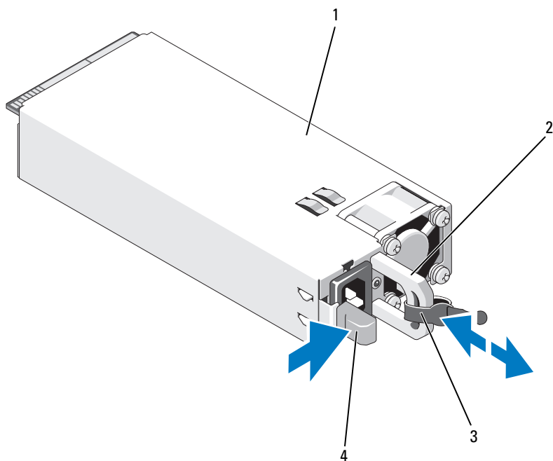
图 3-8. 卸下和安装电源设备
