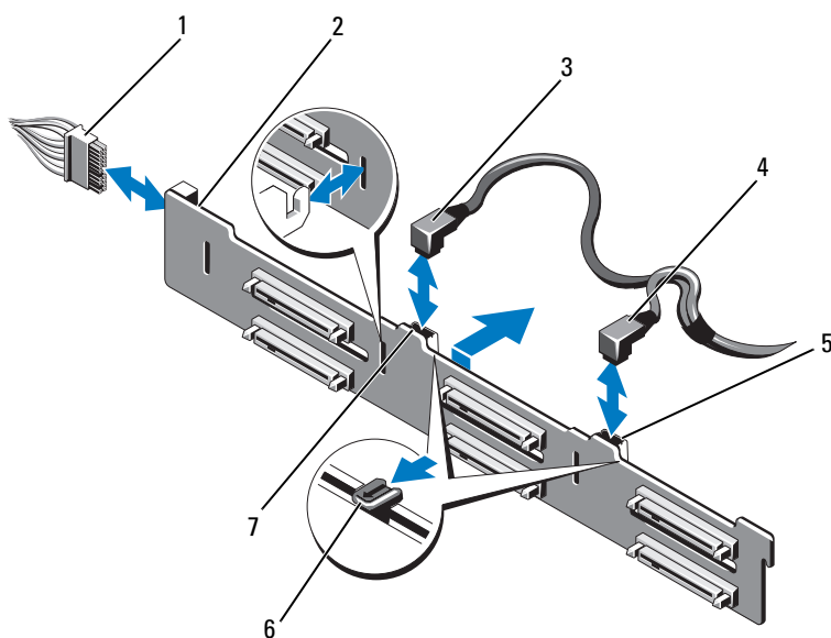
图 3-28. 卸下和安装 SAS 背板
