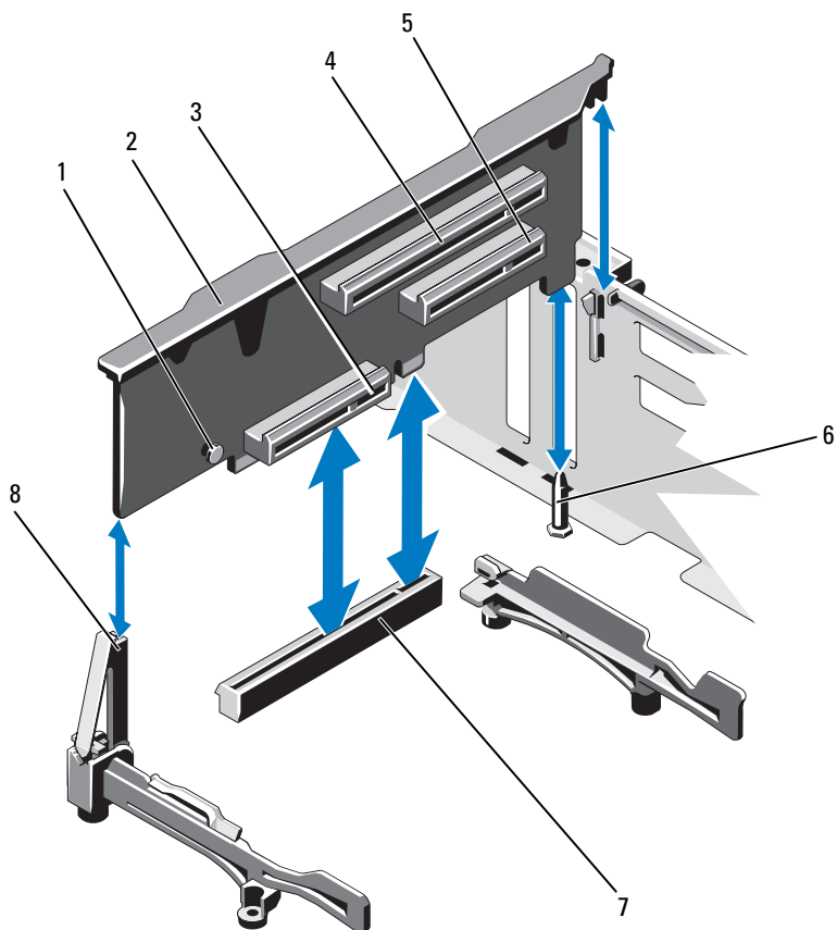
图 3-17. 安装或卸下扩充卡提升板 1
