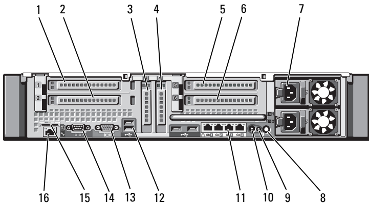
图 1-3. 背面板部件和指示灯
