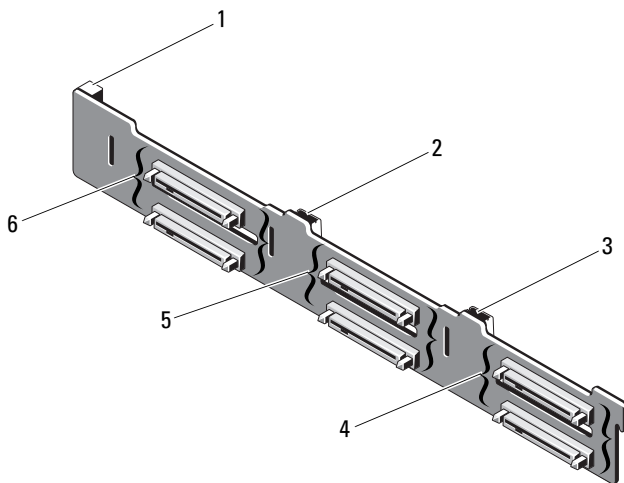
图 6-2. SAS 背板连接器
