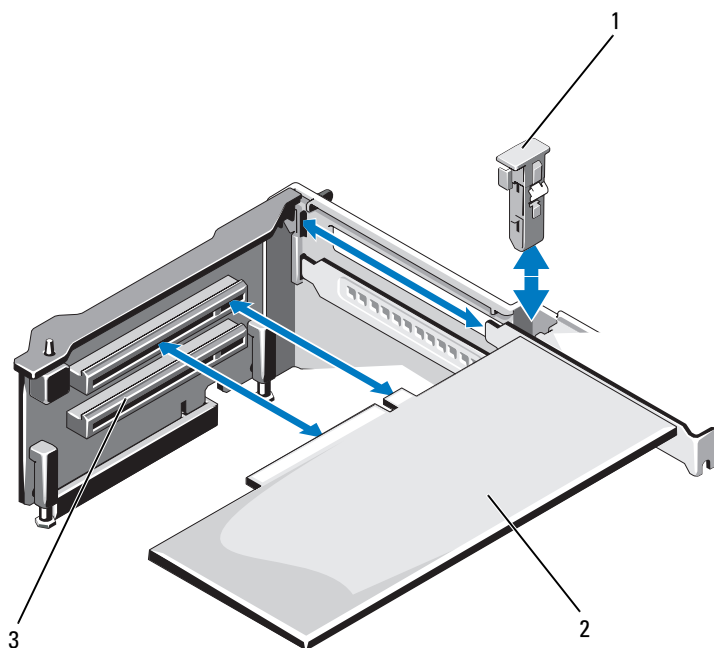
图 3-16. 安装和卸下扩充卡
