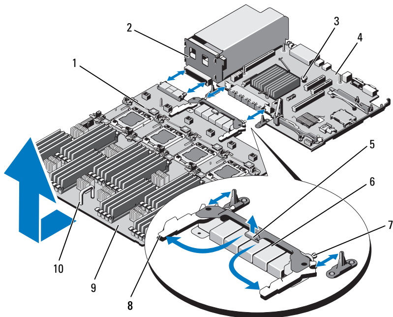
图 3-31. 卸下和安装系统板
