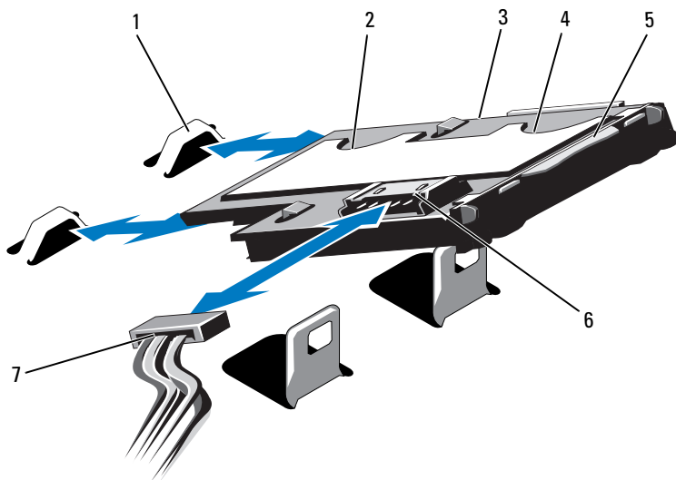
图 3-22. 卸下或安装内部双 SD 模块
