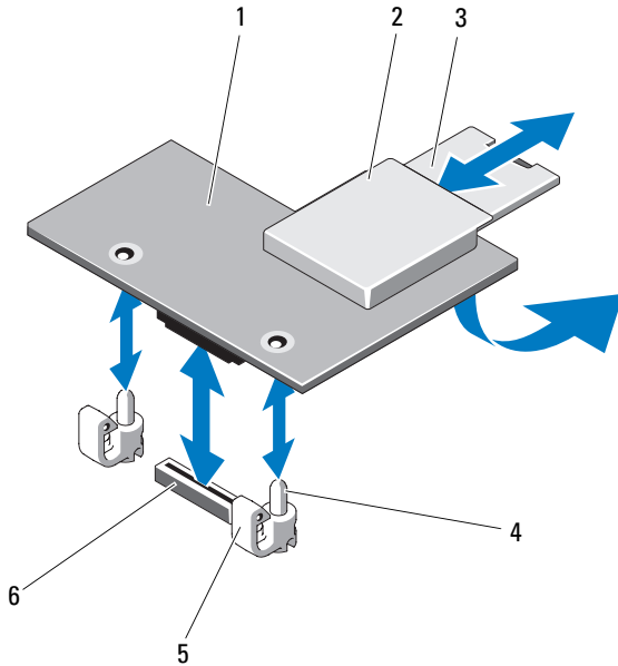
图 3-19. 安装或卸下 iDRAC6 Enterprise 卡（可选）
