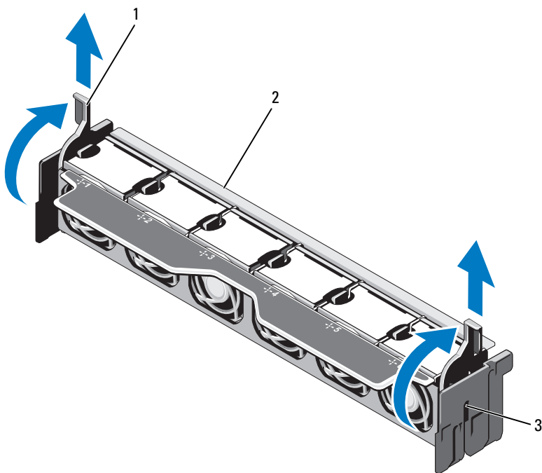
图 3-13. 卸下和安装冷却风扇部件
