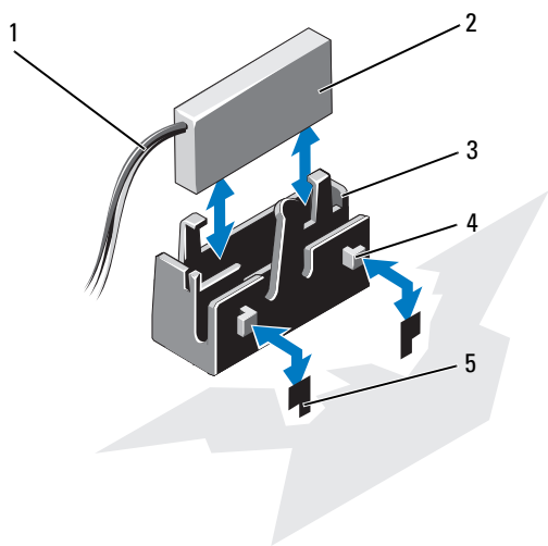
图 3-21. 卸下或安装 RAID 电池
