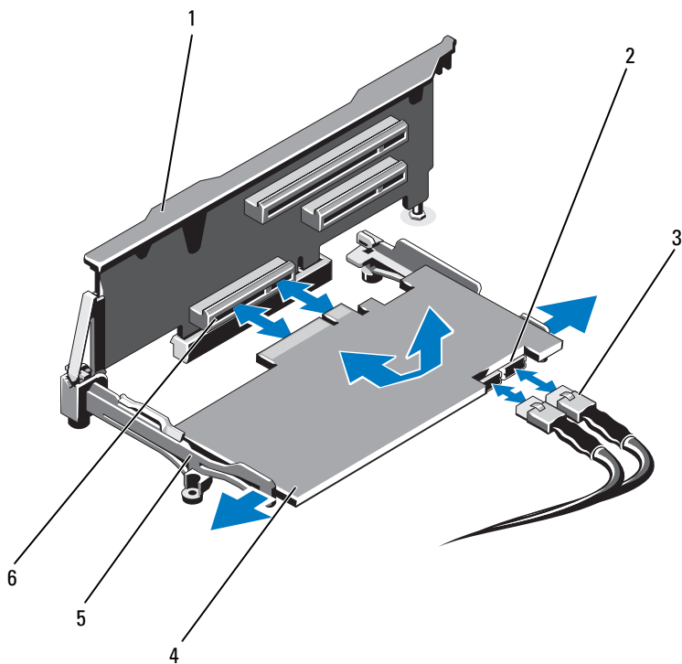
图 3-20. 安装集成存储控制器卡
