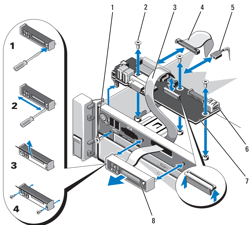
图 3-30. 卸下和安装控制面板显示模块
