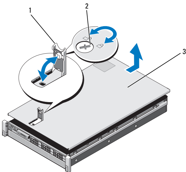
图 3-3. 打开与合上系统护盖
