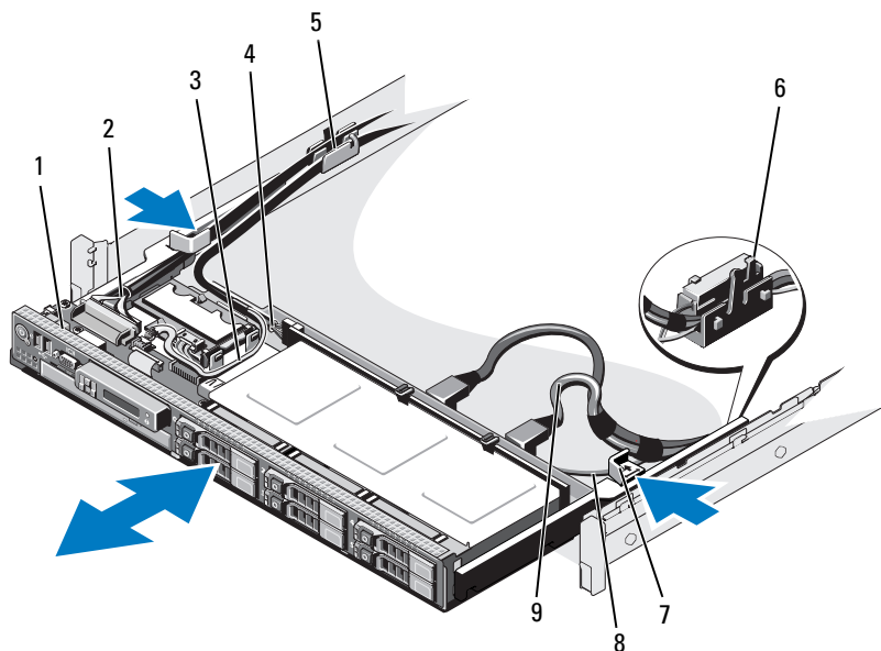
图 3-10. 前机箱部件
