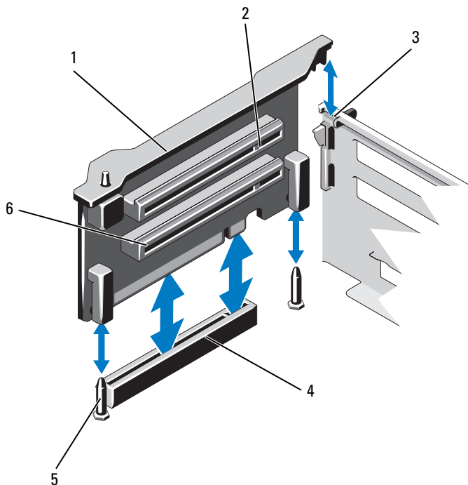
图 3-18. 安装或卸下扩充卡提升板 2
