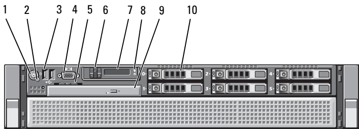
图 1-1. 前面板部件和指示灯
