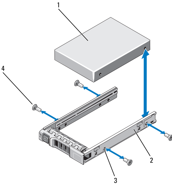
图 3-6. 从硬盘驱动器托盘中卸下热插拔硬盘驱动器或将热插拔硬盘驱动器安装到硬盘驱动器托盘中
