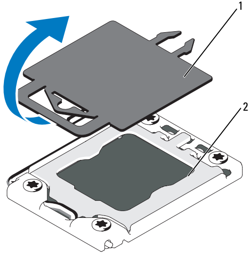
图 3-25. 卸下处理器插槽中的护盖
